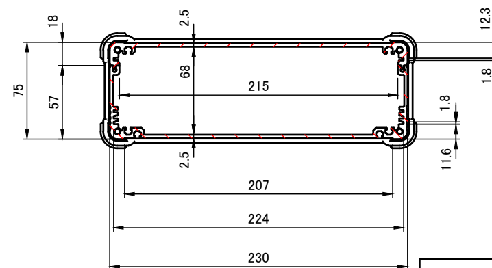
A-A (1:4)
