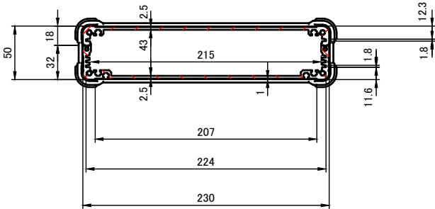
A-A ( 1 : 5 )
