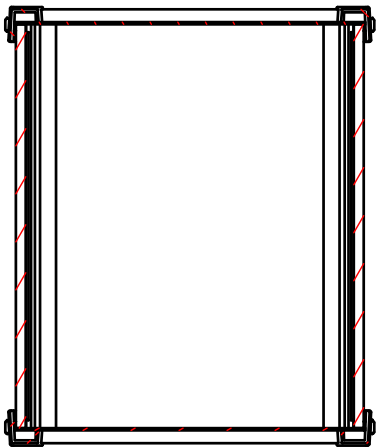
D-D ( 1 : 5 )
