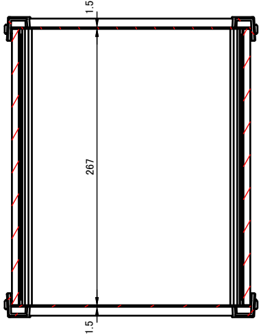
C-C ( 1 : 5 )
