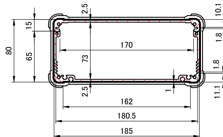
A-A (1:3)
