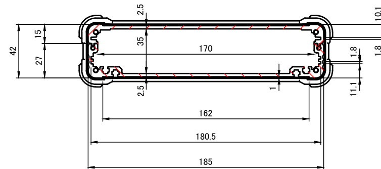
A-A (1:3)
