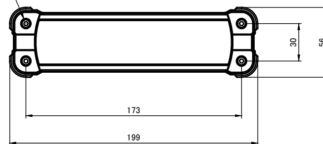
A-A (1:3)
