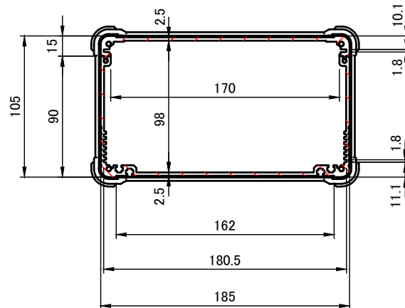
A-A (1:4)
