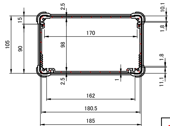
A-A ( 1 : 4 )
