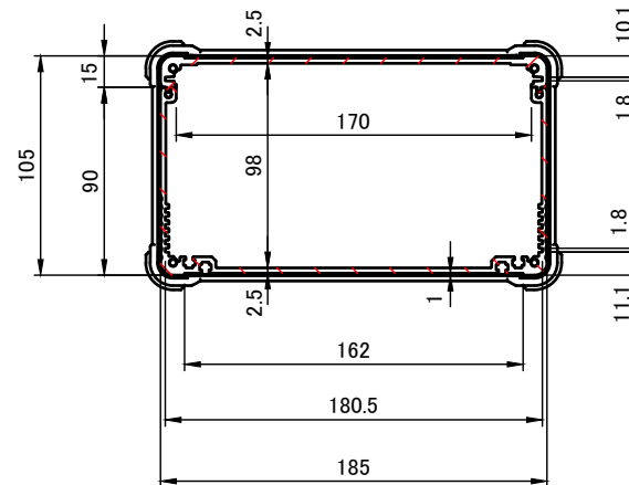
A-A (1:4)
