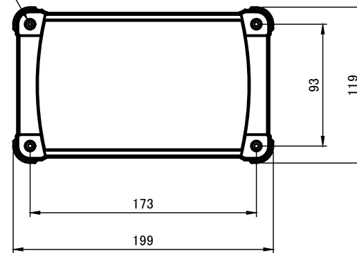
A-A (1:4)
