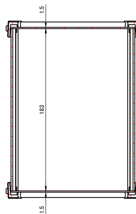
C-C ( 1 : 2.5 )
