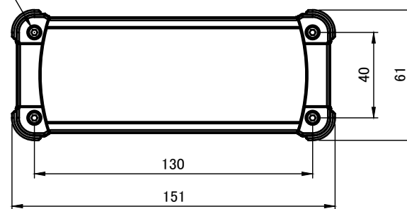
A-A ( 1 : 2.5 )
