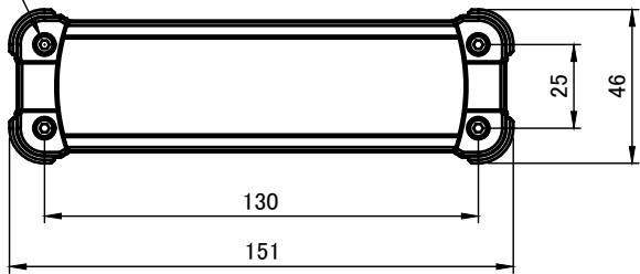
A-A ( 1 : 2.5 )
