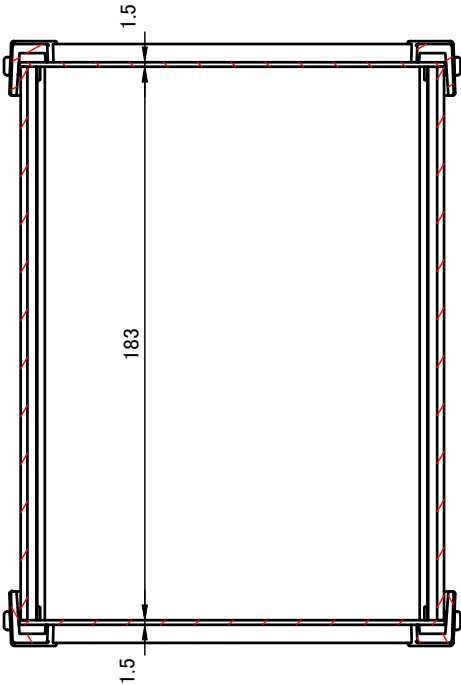
C-C ( 1 : 2.5 )
