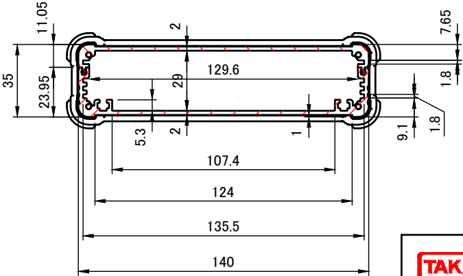
A-A ( 1 : 2.5 )
