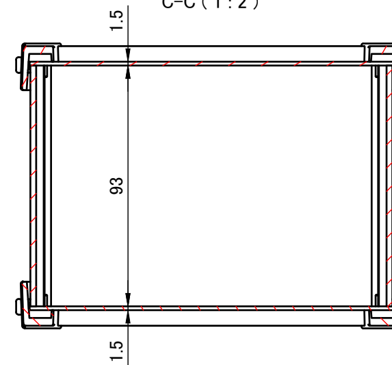
C-C (1:2)
