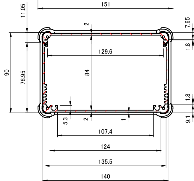
A-A (1:2.5)
