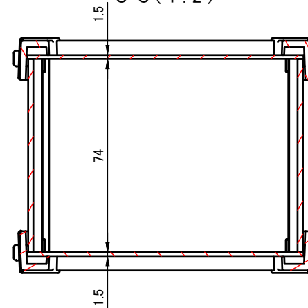
C-C (1:2)
