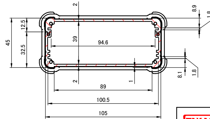
A-A ( 1:2 )
