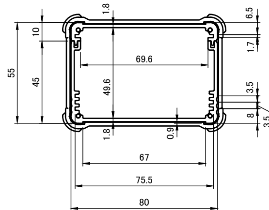
A-A (1:2)
