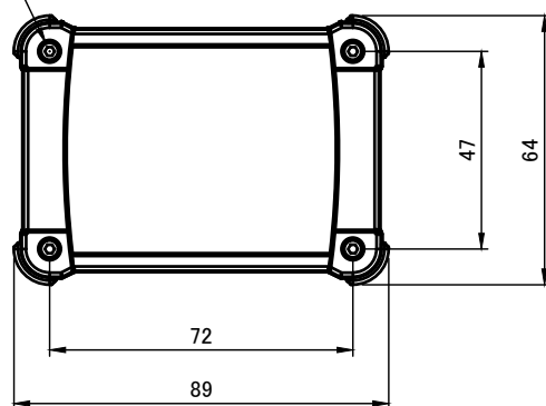
A-A (1:2)
