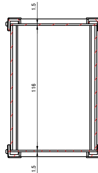
D-D (1:2)
