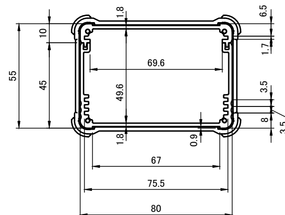
A-A (1:2)
