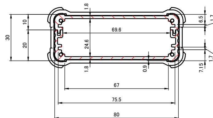
A-A ( 1 : 1.5 )
