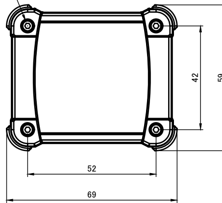
A-A (1:1.5)
