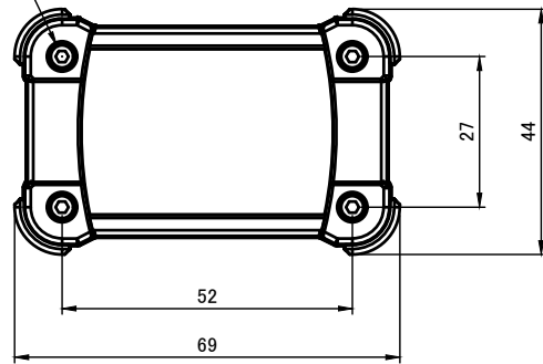
A-A (1:1.5)
