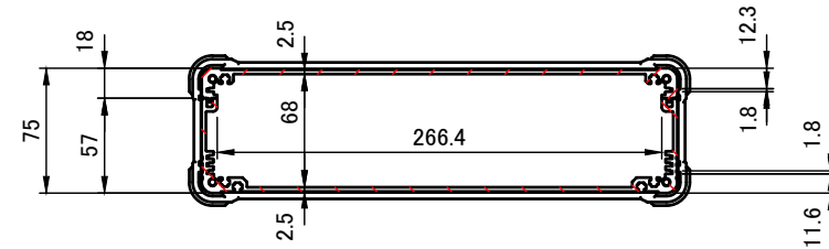
A-A (1:5)
