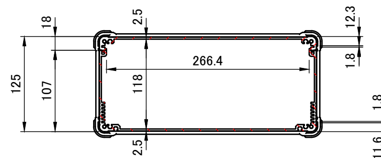
A-A (1:5)
