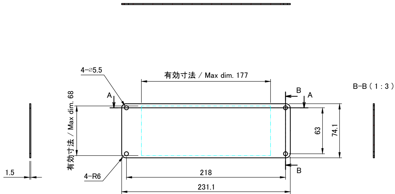
A-A ( 1 : 3 )
