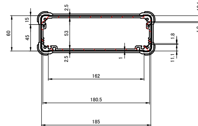
A-A ( 1 : 4 )
