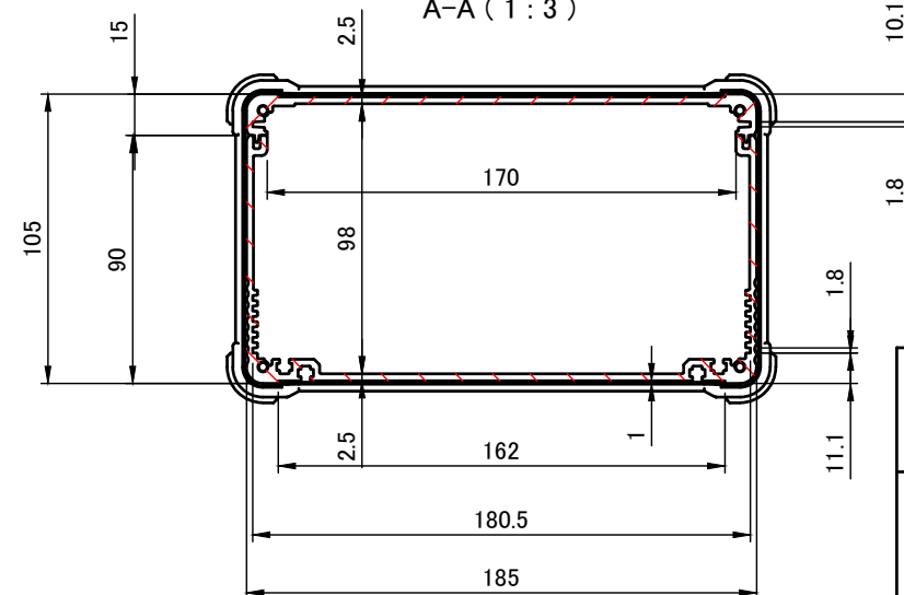
A-A (1:3)
