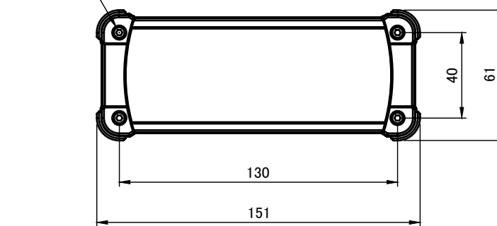
A-A ( 1 : 2.5 )
