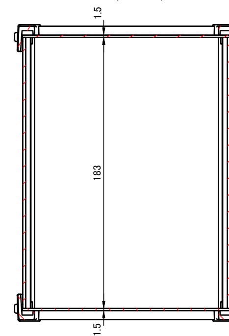
D-D ( 1 : 2.5 )
