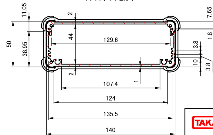
A-A ( 1 : 2.5 )
