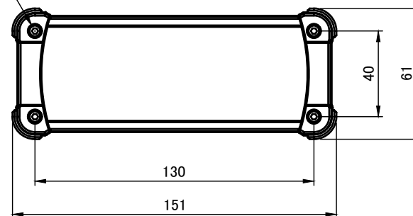
A-A ( 1 : 2.5 )
