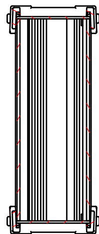
B-B ( 1 : 2.5 )
