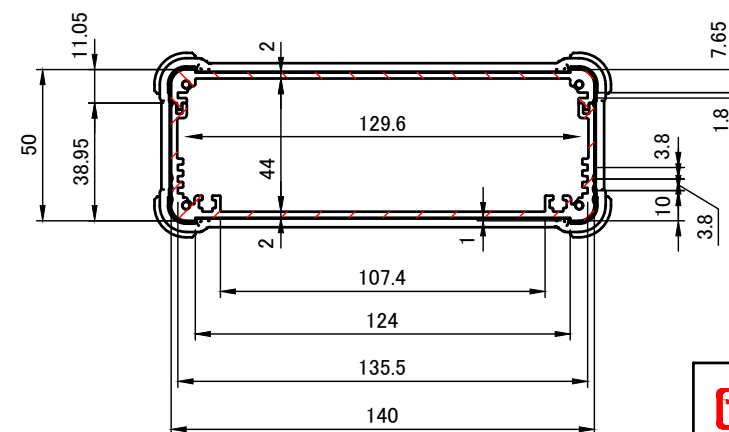
A-A ( 1 : 2.5 )
