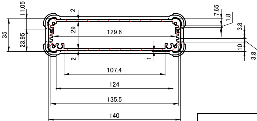
A-A ( 1 : 2.5 )
