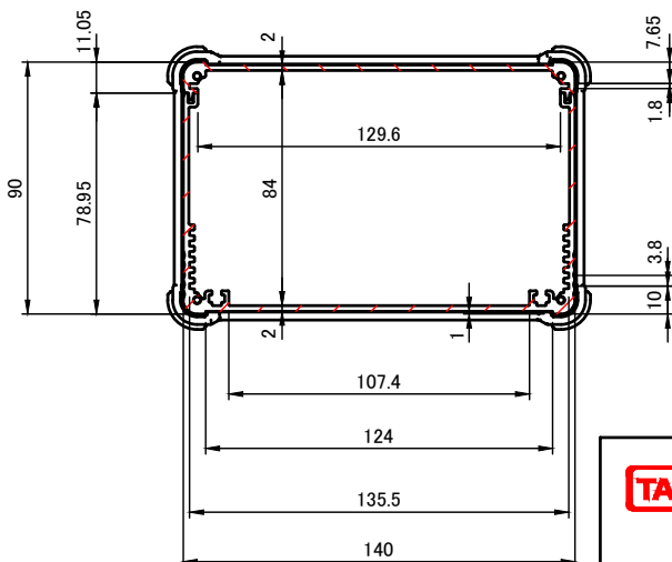
A-A ( 1 : 3 )
