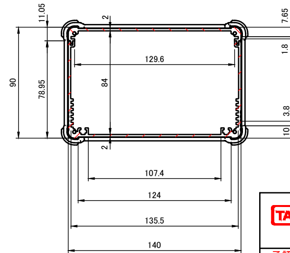
A-A (1:3)
