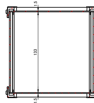
D-D (1:3)
