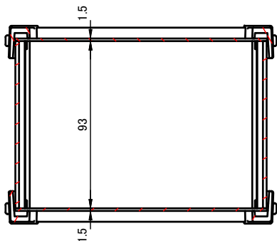
D-D (1:3)
