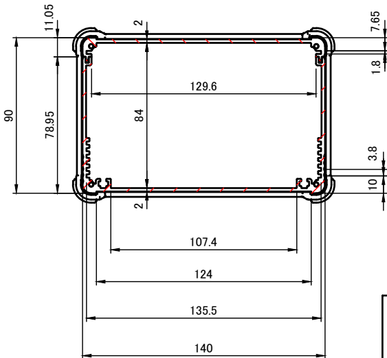
A-A (1:3)
