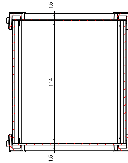
D-D (1:2)
