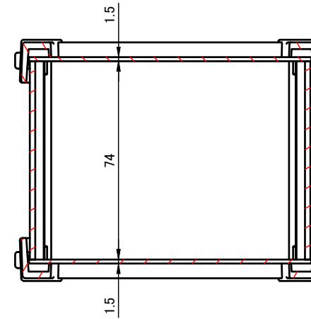
D-D (1:2)
