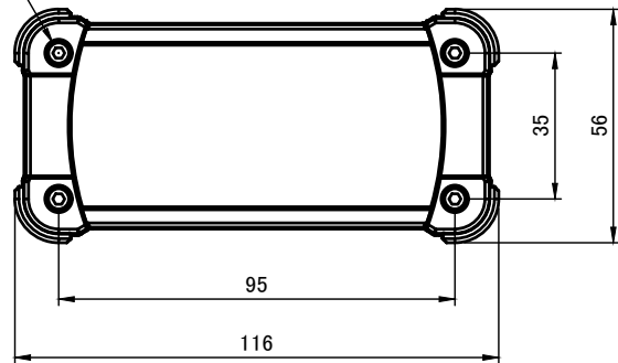
A-A (1:2)
