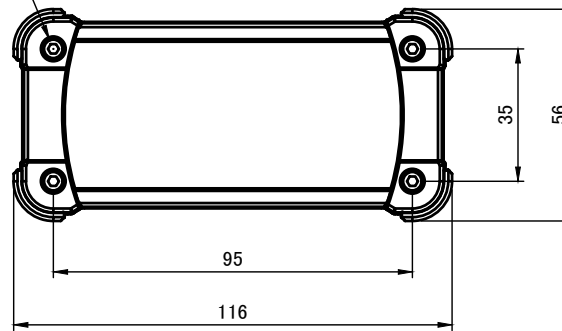
A-A (1:2)
