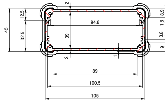
A-A (1:2)
