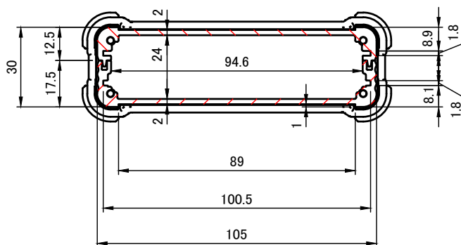
A-A (1:2)
