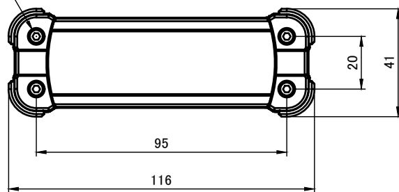
A-A (1:2)
