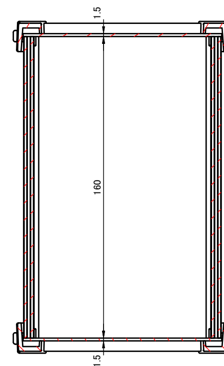
D-D (1:2)
