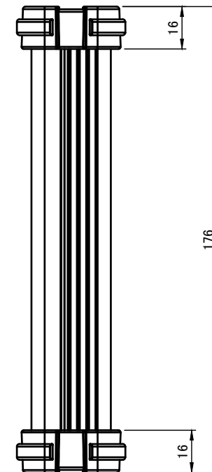
D-D (1:2)
