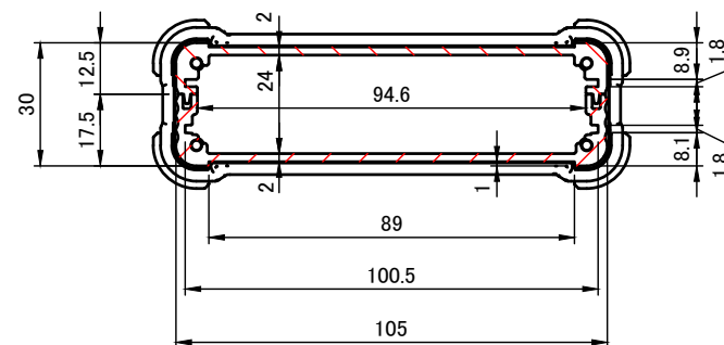
A-A (1:2)
