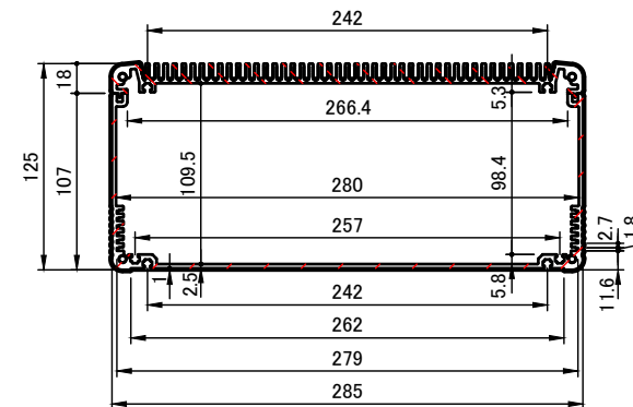
A-A (1:5)
