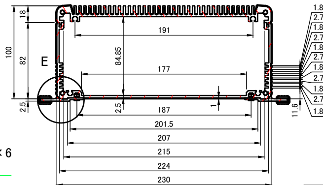
A-A (1:4)
