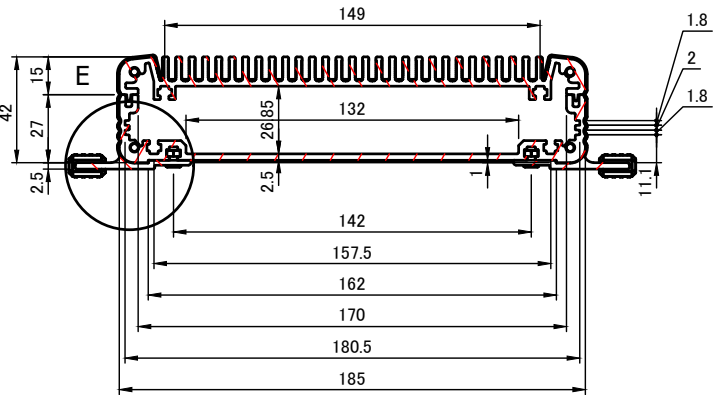
A-A ( 1 : 3 )
