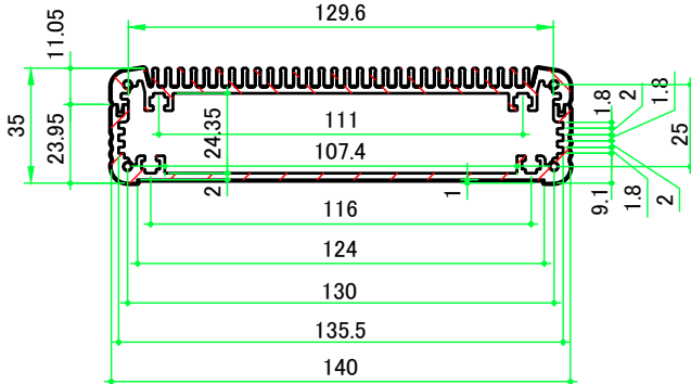
A-A ( 1 : 2.5 )
