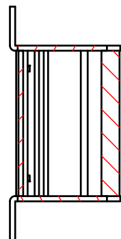
B-B (1:2)
