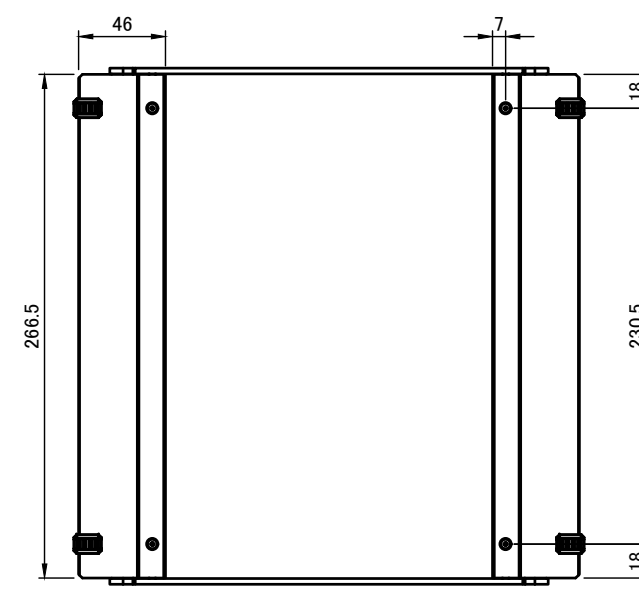
D-D (1:4)
