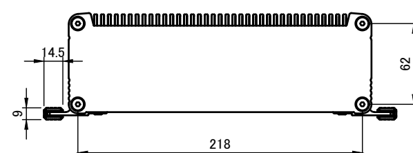
A-A (1:4)
