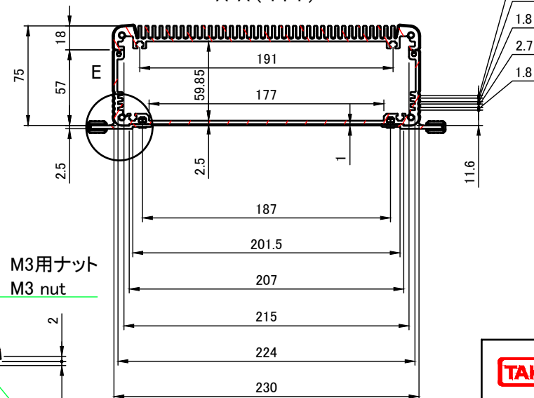
A-A (1:4)
