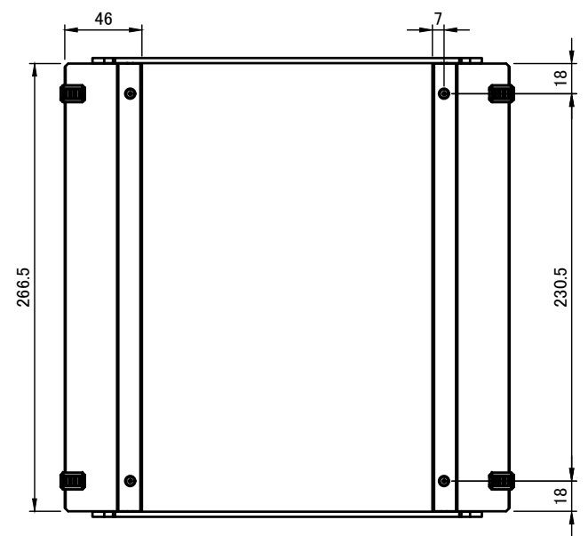
D-D (1:4)
