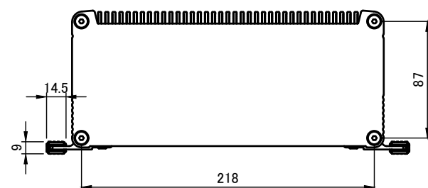
A-A (1:4)
