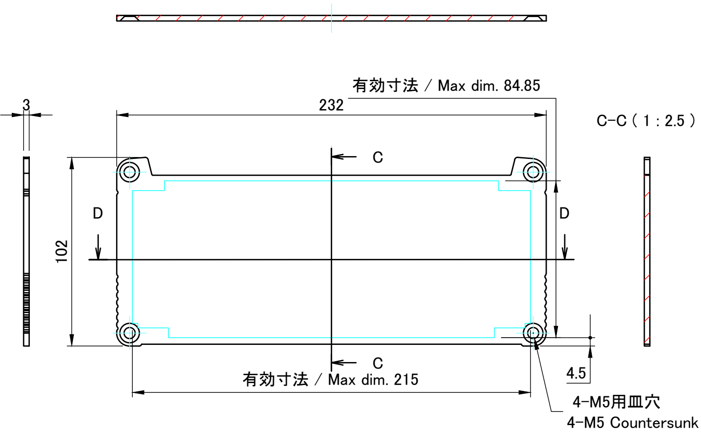
D-D ( 1 : 2.5 )
