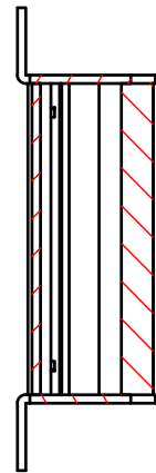
B-B (1:2)
