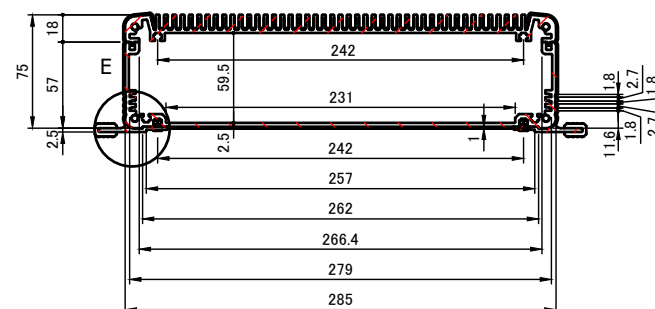
A-A (1:5)
