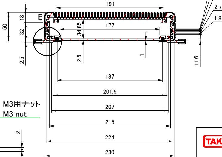
A-A ( 1 : 4 )
