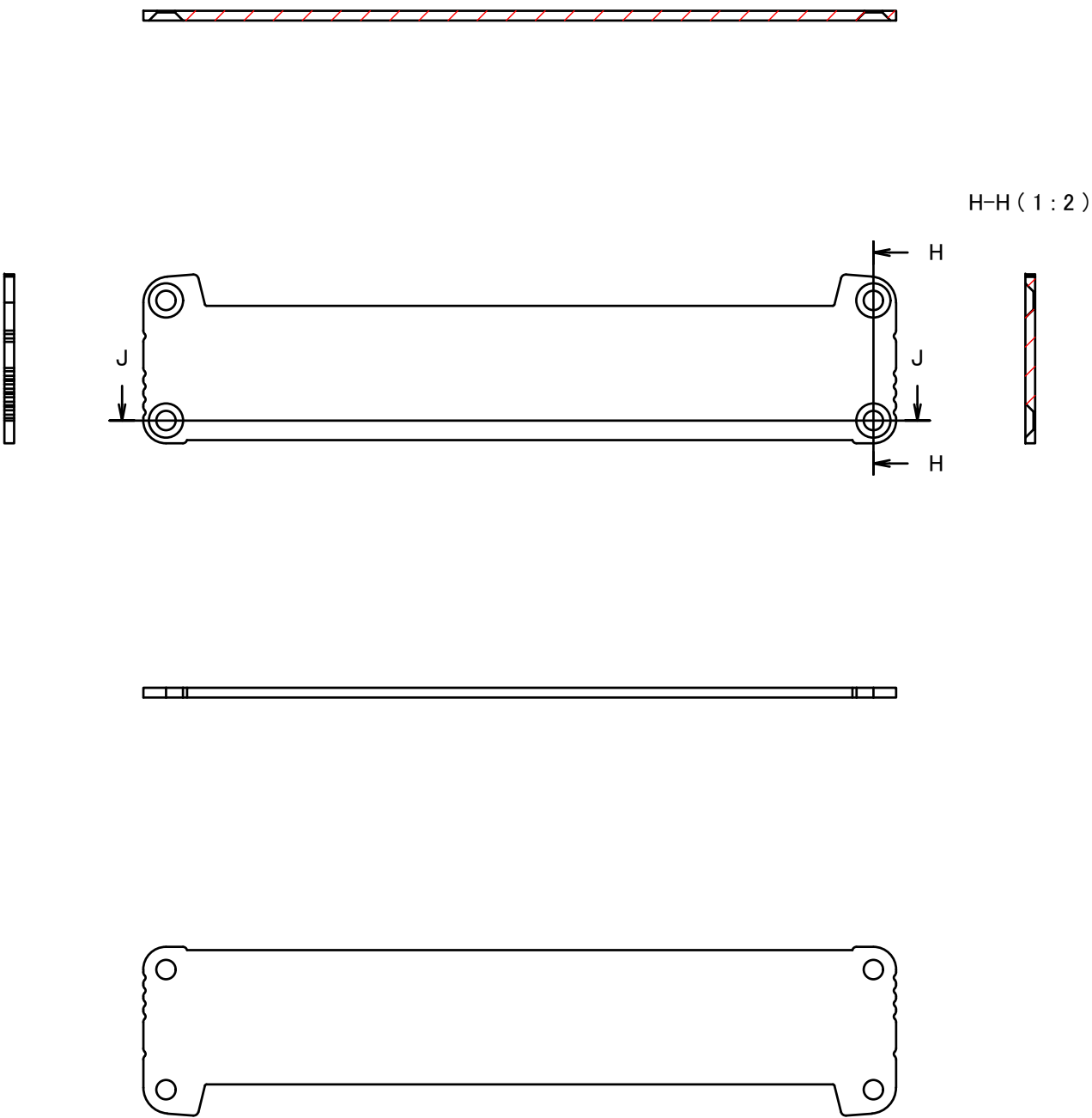
J-J ( 1 : 2 )
