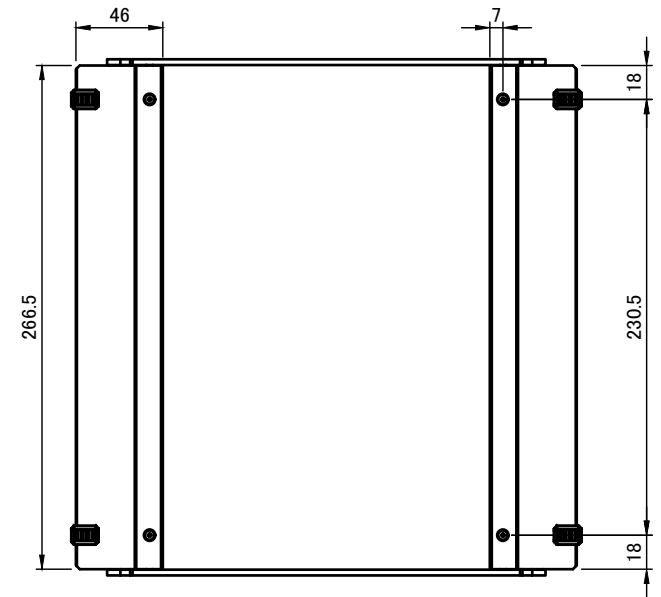
D-D (1:4)
