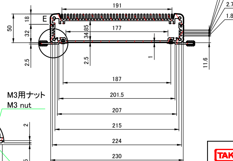
A-A (1:4)
