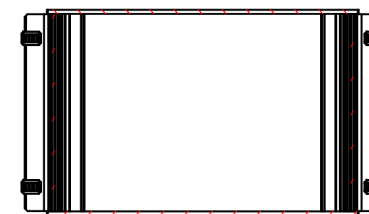
D-D (1:4)
