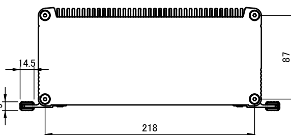
A-A (1:4)
